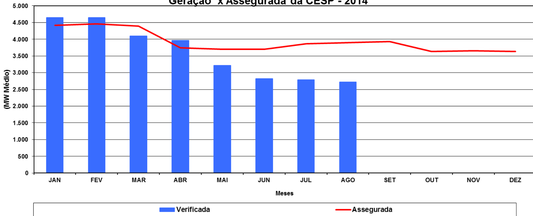
Geração x Assegurada da CESP - 2014
